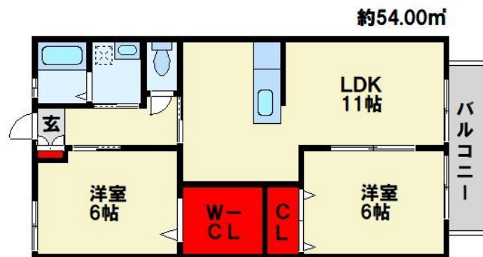
【間取り図】
