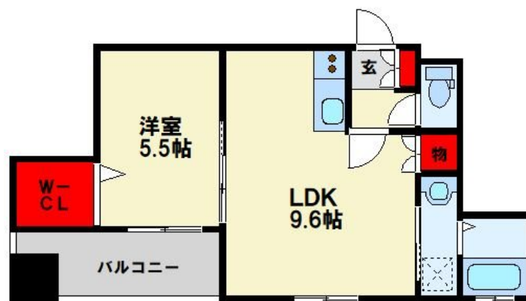
【間取り図】
